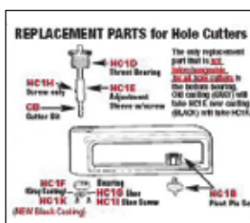
ΑΝΤΙΚΑΤΑΣΤΑΣΗ ΤΡΥΠΑΝΙΟΥ
