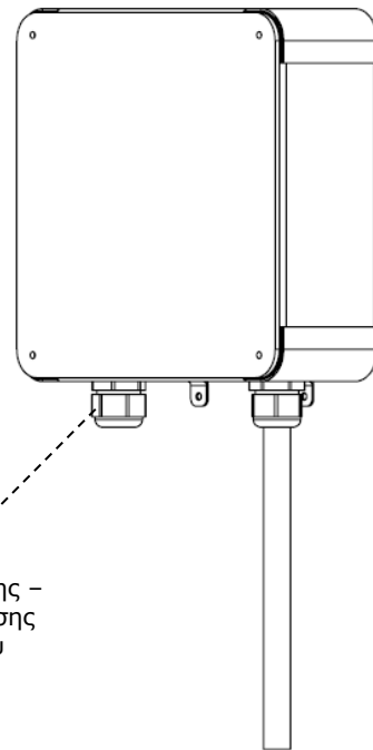
Σχήμα 4 - Το παροχικό καλώδιο οδηγείται μέσα από τον στυπιοθλύπτη στο εσωτερικό του φορτιστή
