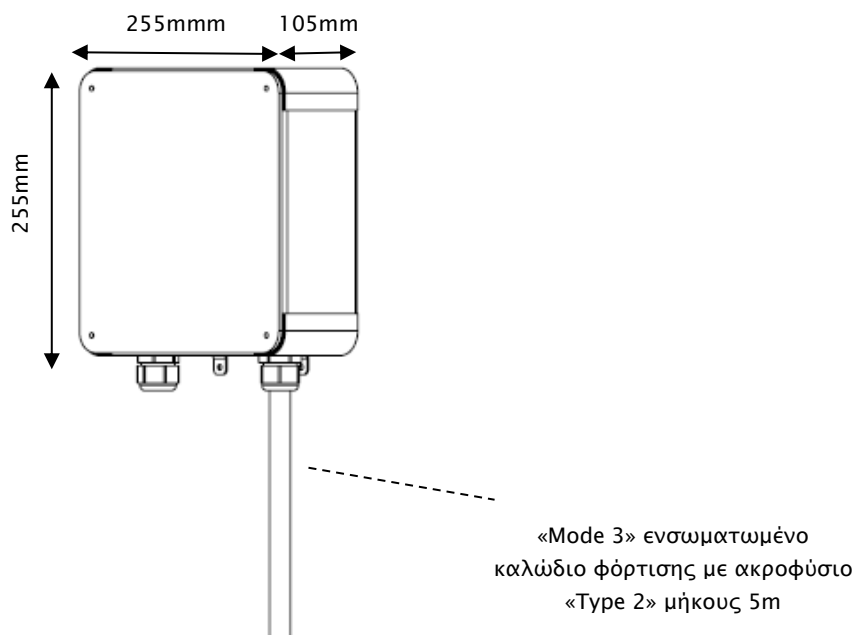
Σχήμα 1: Διαστάσεις φορτιστή UCS1 22KW
