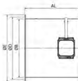
TGT long casing
